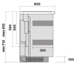
Widok z boku z ewentualnymi szufladami
